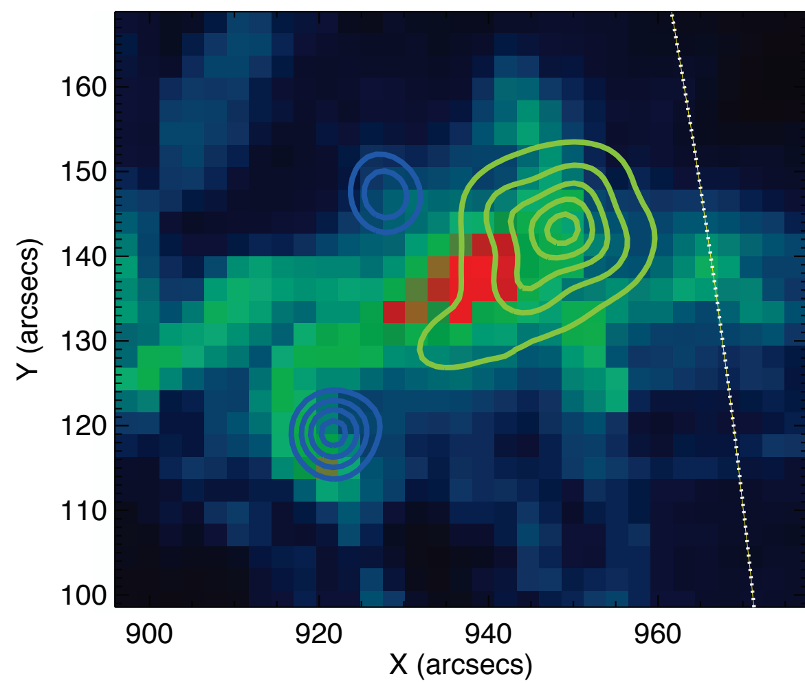
SOHO EIT 195 3-Nov-2003 09:48:10.832 UT
